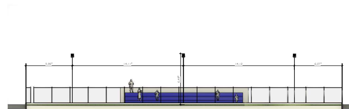
④ CORTE LATERAL 2 1 : 100
