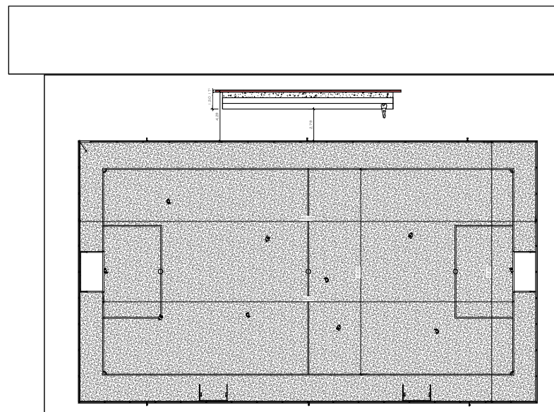
② TÉRREO Copilar 1 1 : 100
