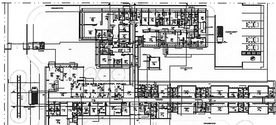
FIGURA 5: PLANTA BAIXA DO HOSPITAL
