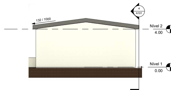
5 Corte 3 1 : 100
