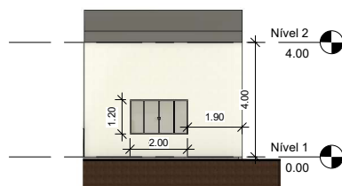
3 Corte 1 1 : 100
