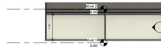
3 Corte 2 1 : 100
