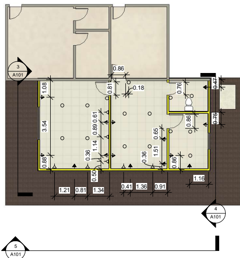
1 Nível 1 1 : 100
