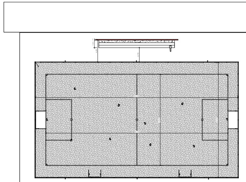
2 - TÉRREO Copiar 1 1 : 100
